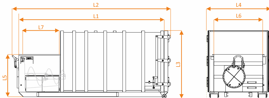
SPB LM 23 SPS met speciale opbouw (incl. kijkvenster, ladder en aan de achterzijde scharnierend deksel)
